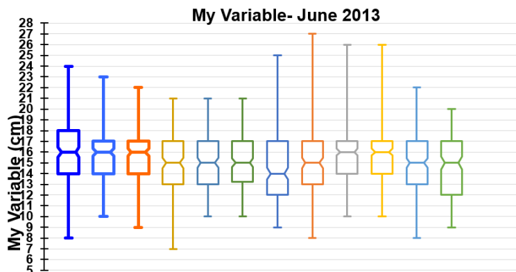
Figura 7 – Identificação de problemas usando Box Plot.
