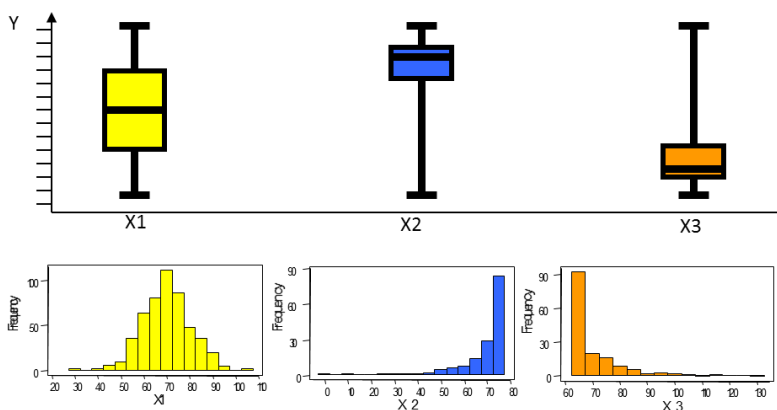
Figura 2 – Comparação do Box Plot com Histograma.
