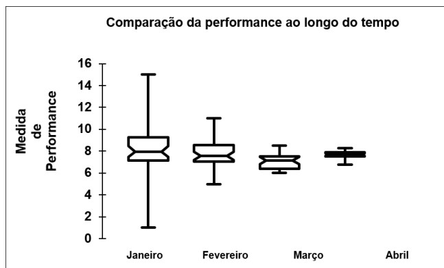
Figura 6 – Comparação de performance usando Box Plot.
