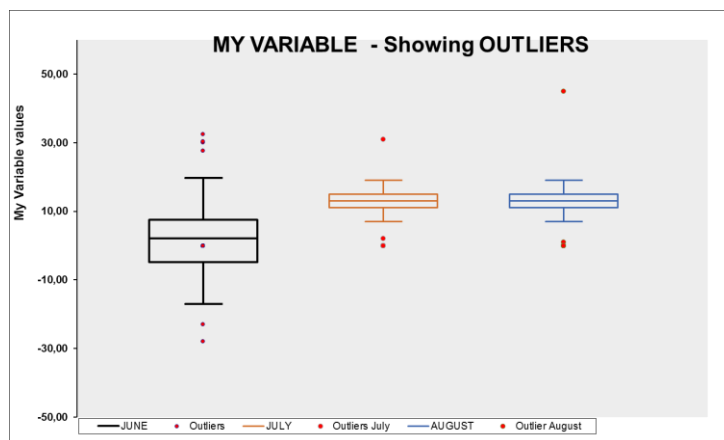
Figura 8 – Identificação de Outliers usando Box Plot.
