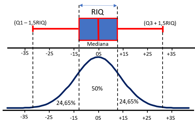
Figura 9 – Racional da identificação de Outliers usando Box Plot.
