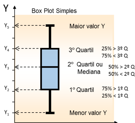
Figura 1 – Interpretação do Box Plot simples.
