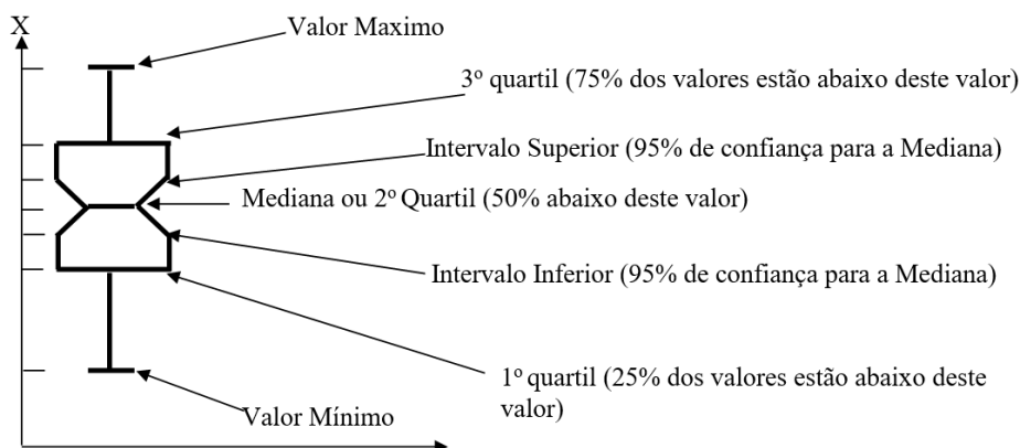
Figura 4 – Interpretação do Box Plot chanfrado.
