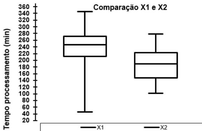
Figura 3 - Comparação de variáveis com Box Plot.
